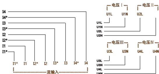
图一 交流单相电压电流测量接线方式
