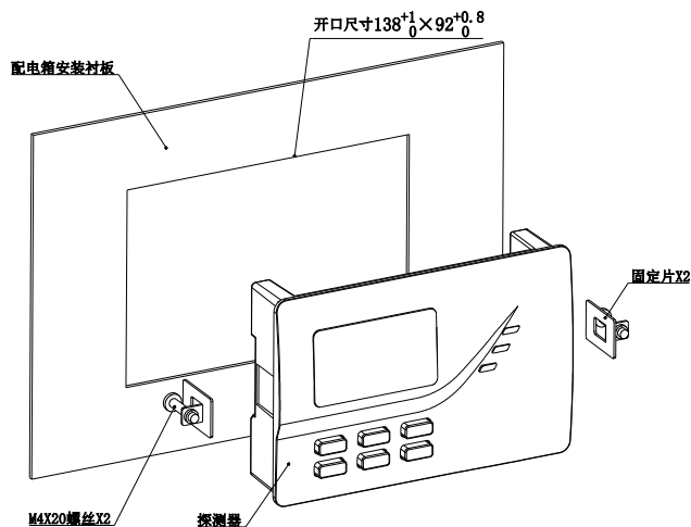
图 8-a 嵌装于箱体面板上
