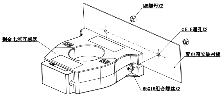
图 13 开口式圆孔型剩余电流互感器安装过程分解图
