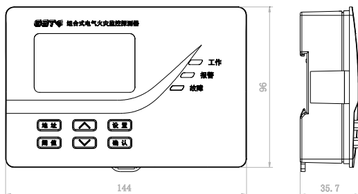
图 1 探测器信号处理单元外形示意图
