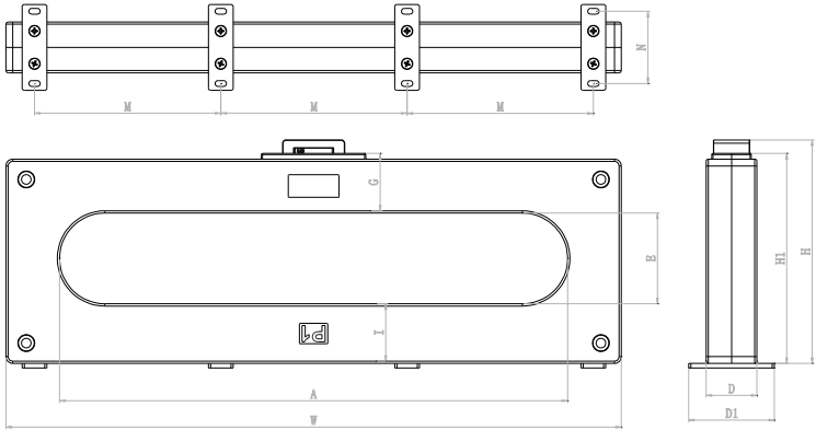
图 5 DH-GST-N2200-F-2000 剩余电流互感器外形示意图
