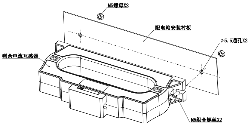
图 10 闭口方孔型剩余电流互感器安装过程分解图
