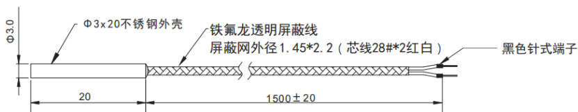
图 7 测温传感器外形图
