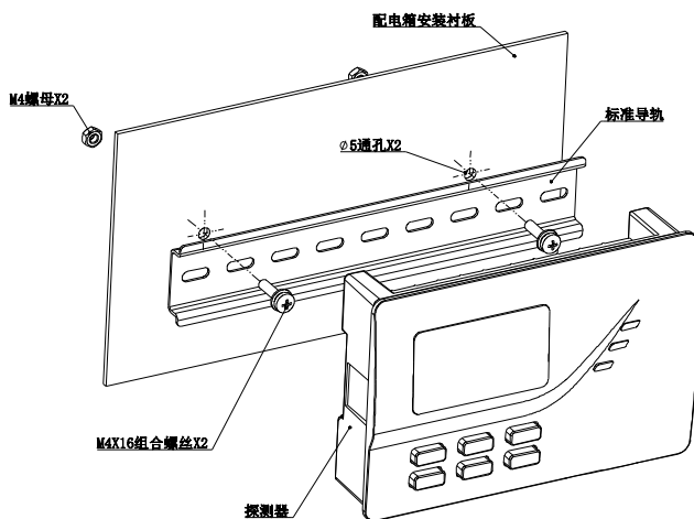
图 8-b 导轨安装
