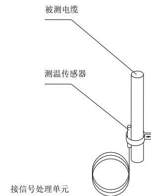
图 14 测温传感器安装图
