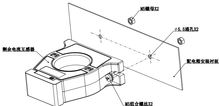
图 9 闭口圆孔型剩余电流互感器安装过程分解图
