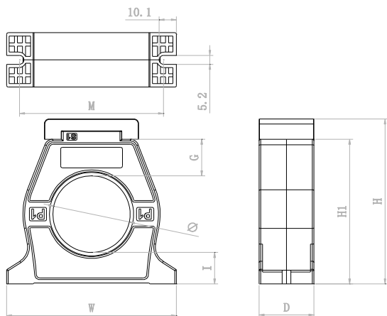
图 2 闭口式圆孔型剩余电流互感器外形示意图
