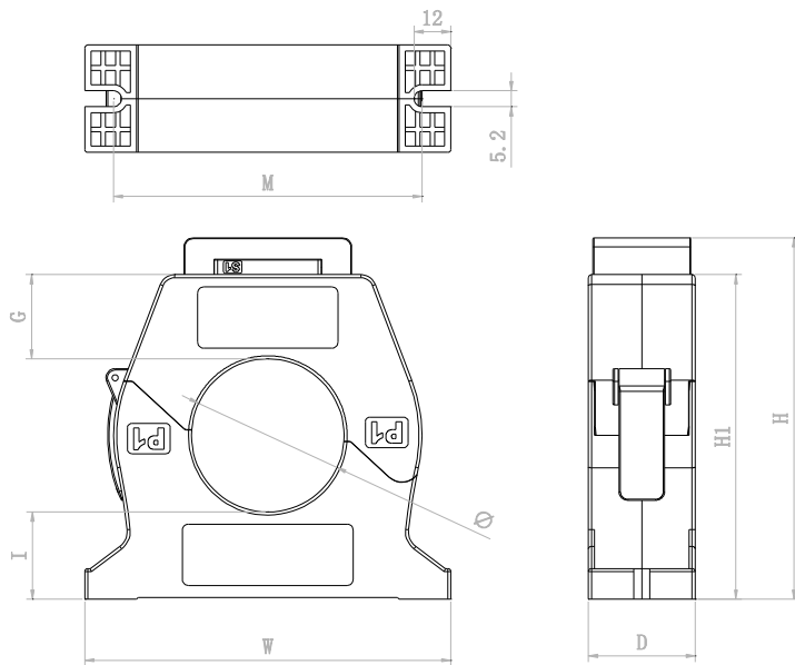
图 6 开口式圆孔型剩余电流互感器外形示意图
