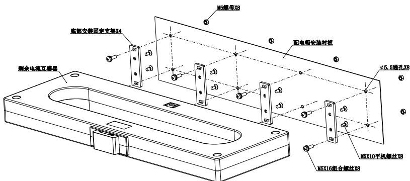
图 12 DH-GST-N2200-F-2000 剩余电流互感器安装过程分解图
