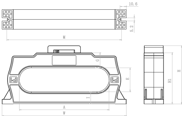
图 3 闭口式方孔型剩余电流互感器外形示意图
