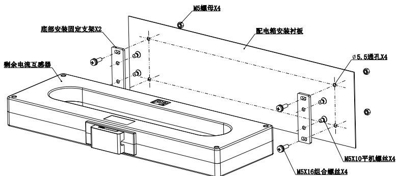
图 11 DH-GST-N2200-F-1000 剩余电流互感器安装过程分解图
