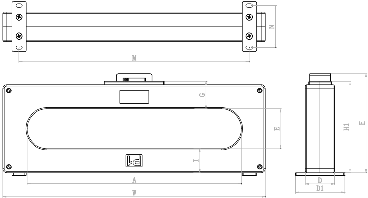
图 4 DH-GST-N2200-F-1000 剩余电流互感器外形示意图
