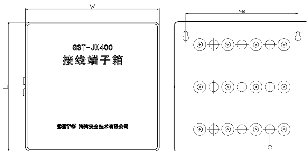
图 1 接线端子箱外形示意图
