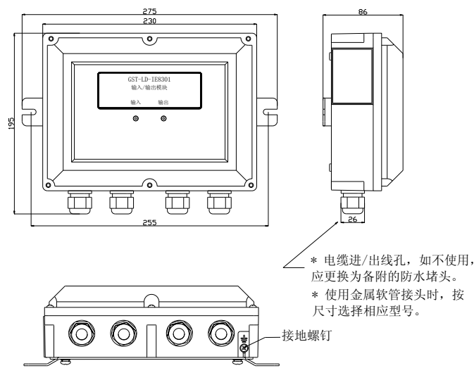
图 1 外形示意图
